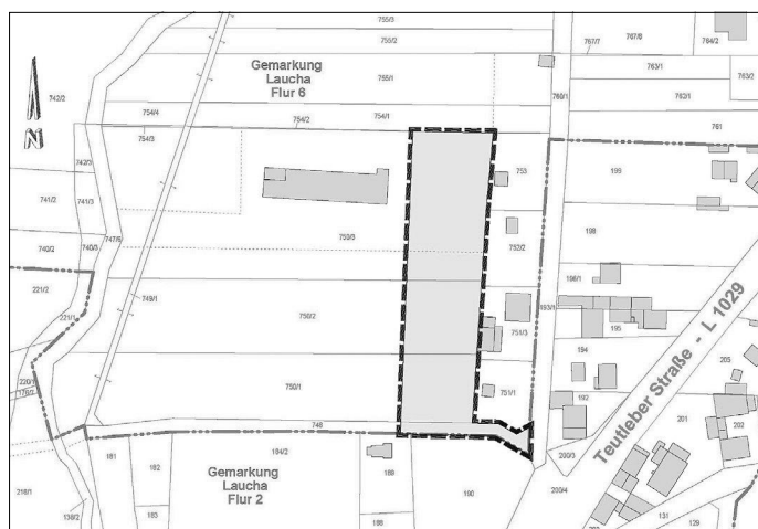
Übersichtslageplan zum Geltungsbereich des Bebauungsplans für die Fläche für den Gemeinbedarf „Gemeindejugendzentrum“ im Ortsteil Laucha
